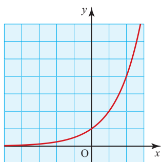
(d) Increasing for all values of x
